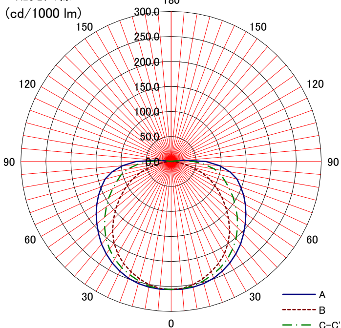
配光曲線
