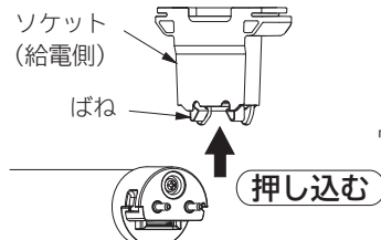
ランプの取り付けかた (図4)
