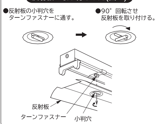
反射板の取り付けかた(図4)
