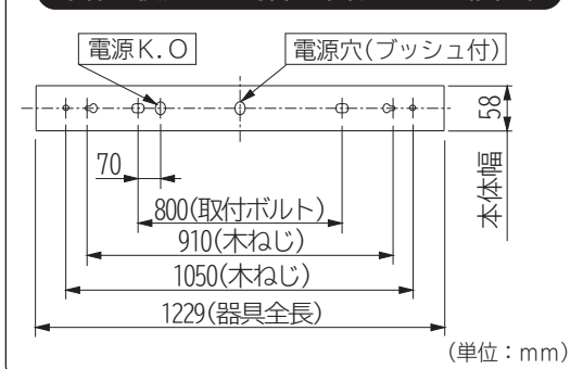
単体で使用する場合の取付ピッチ(図1)
