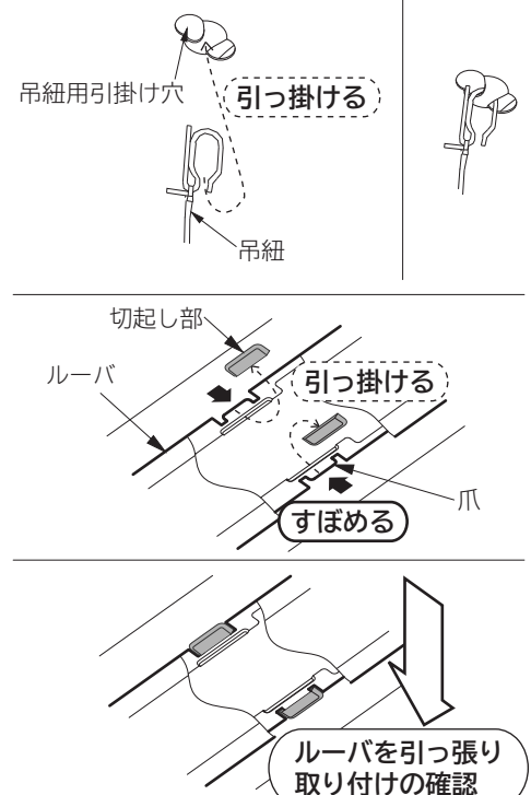
ルーバの取り付けかた (図4)
