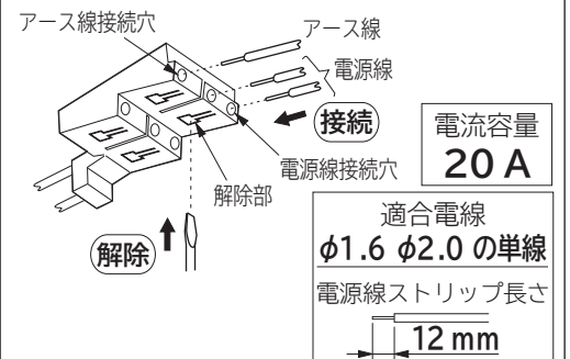
調光端子台の接続と解除 (図3)
