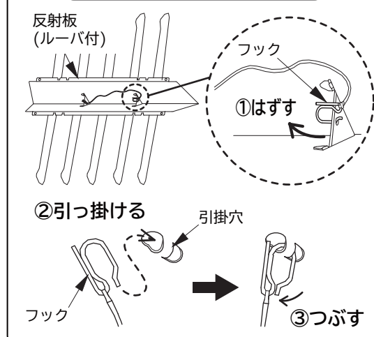
落下防止ひもの取り付け(図4)
