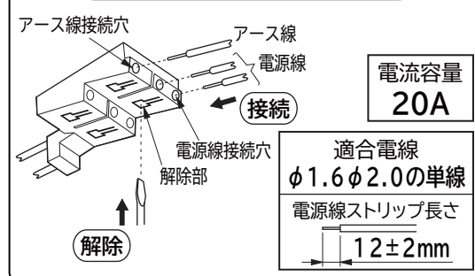
調光端子台の接続と解除(図3)
