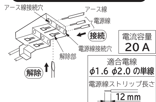
調光端子台の接続と解除 (図3)
