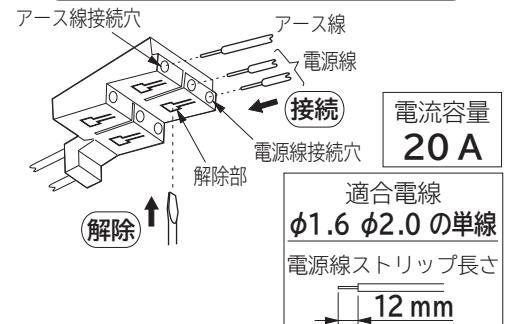
調光端子台の接続と解除 (図3)
