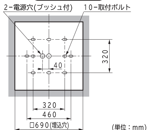
背面取付穴(図1)
