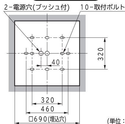
背面取付穴(図1)
