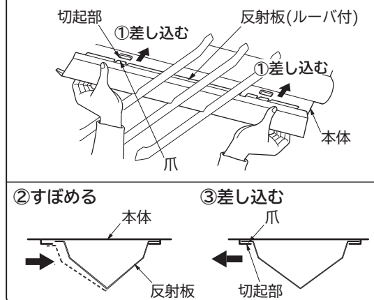
反射板の取り付けかた(図5)
