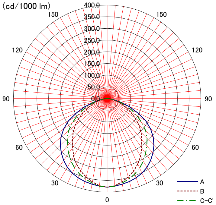
配光曲線
