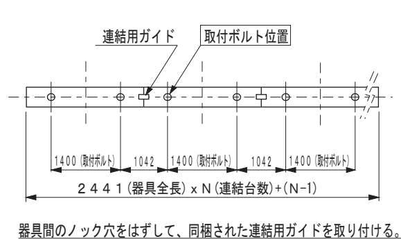
単体N連結する場合の取付ピッチ（図4）
