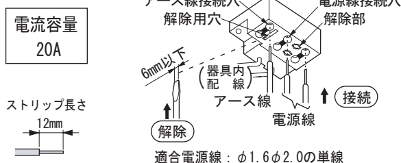
連結端子台の接続と解除（図2）
