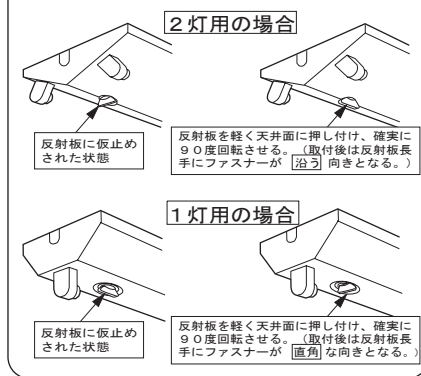
反射板取付方法（図3）
