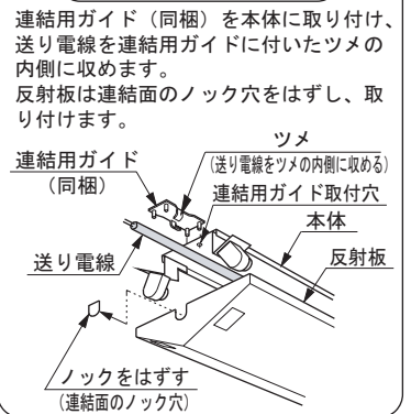
連結のしかた（図5）
