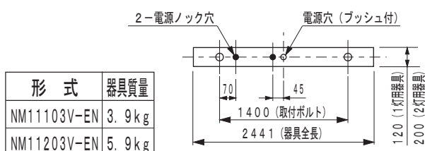
器具質量と背面取付穴（図1）
