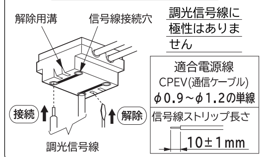
調光端子台の接続と解除(図4)
