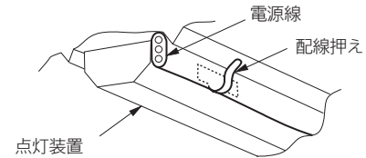
電源端子台の接続と解除 (図2)
