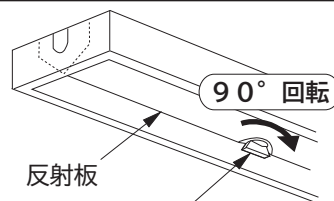
反射板の取り付けかた (図3)
