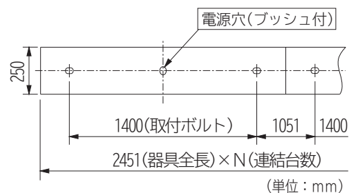
電源線の器具内送り配線を行う場合
