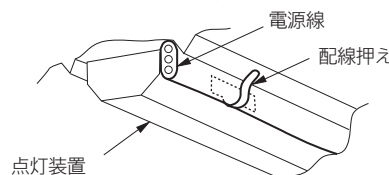
電源端子台の接続と解除 (図2)
