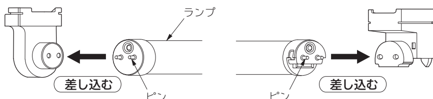
ランプの取り付けかた (図4)
