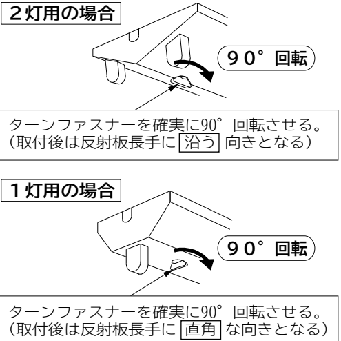
反射板の取り付けかた (図4)
