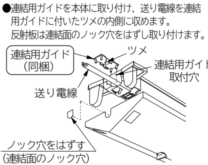
連結端子台の接続と解除 (図3)
