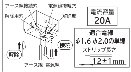
調光端子台の接続と解除(図4)
