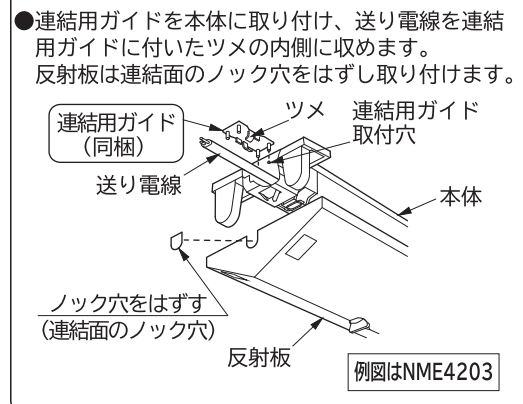
電源端子台の接続と解除(図3)
