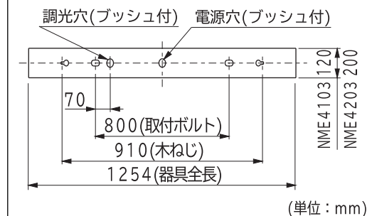
連結のしかた(図2)
