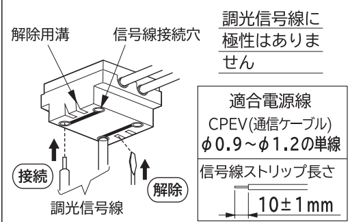
調光端子台の接続と解除(図4)
