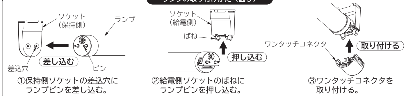
ランプの取り付けかた (図5)
