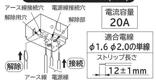
調光端子台の接続と解除(図3)
