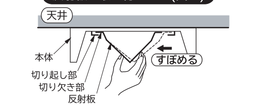
反射板の取り付けかた(図4)
