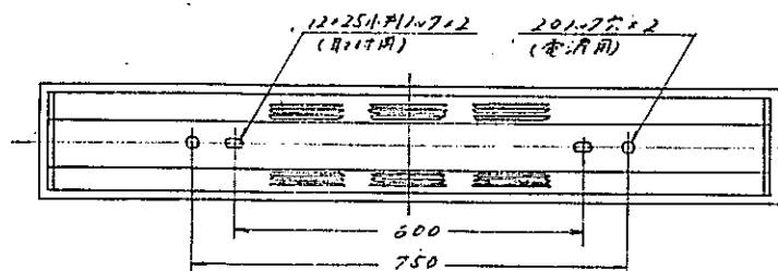
背面寸法図 ( s = \frac{1}{10} )
