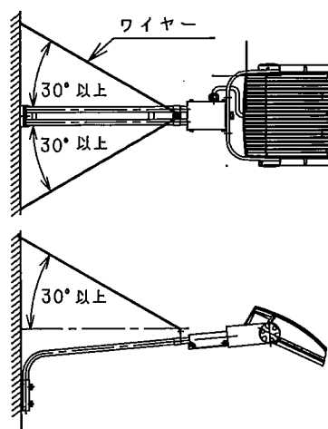
ワイヤーの施工方法
