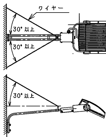
ワイヤーの施工方法
