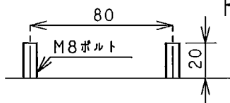
建築物取付ボルト図
