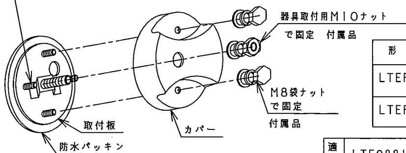
構造物への取付方法
