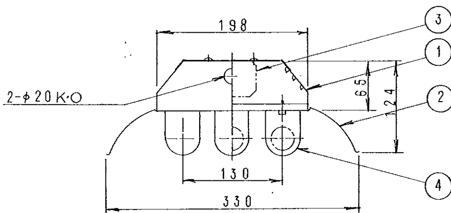
連結金具形式 B-13
