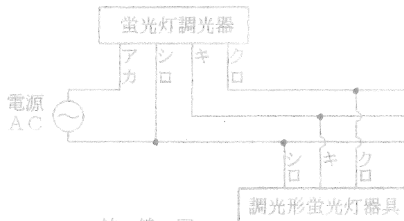
結線図
