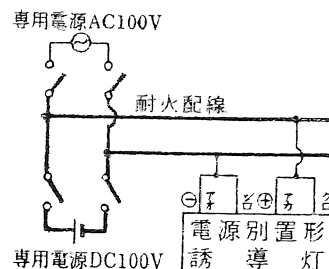
2線配線方式
