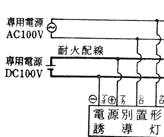
4線配線方式
