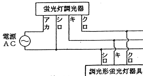
結線図
