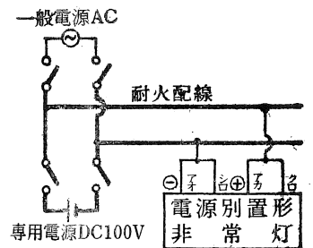
2線配線方式
