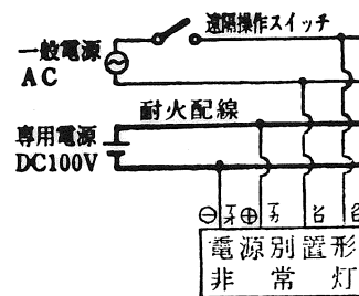
4線配線方式
