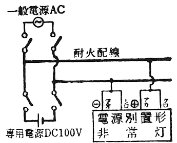
2線配線方式
