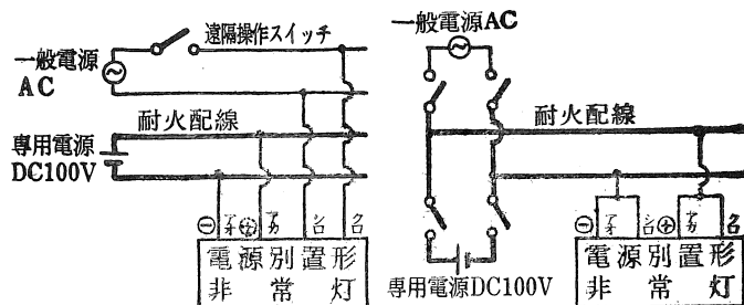
4 線配線方式
