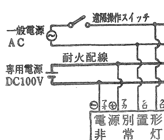
4 線配線方式
