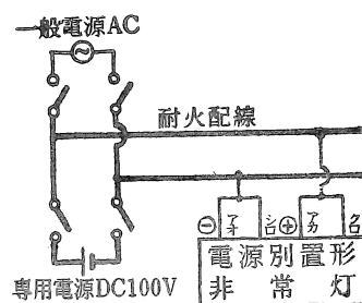
2 線配線方式
