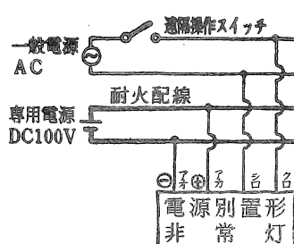
4線配線方式
