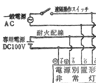
4 線配線方式
