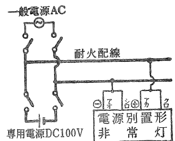
2線配線方式
