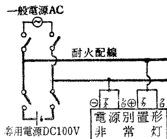
2 線配線方式
