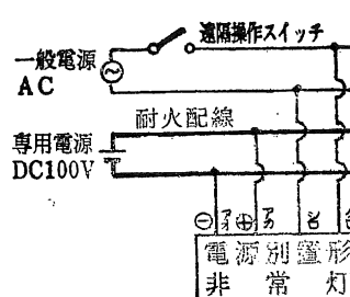
4線配線方式
