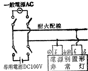
2線配線方式
