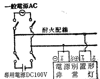
2線配線方式
