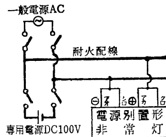
2 線配線方式
