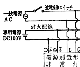
4 線配線方式
