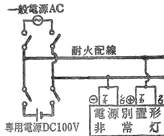
2 線配線方式
