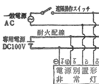
4 線配線方式
