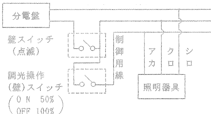
結線図
