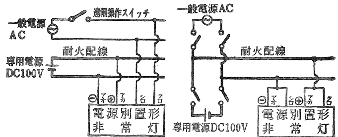
4 線配線方式
