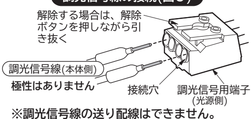
調光信号線の接続(図5)
