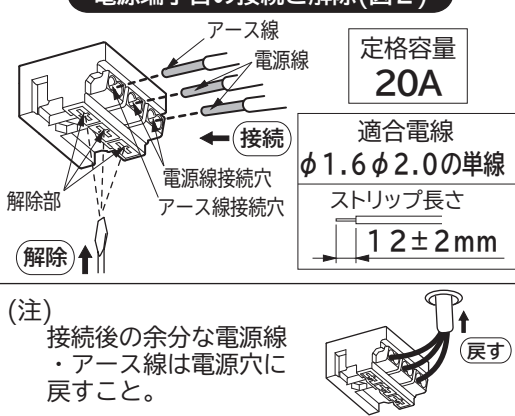
取付パネの取り付け(図3)
