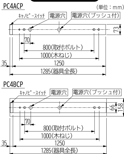
背面取付穴 (図1)
