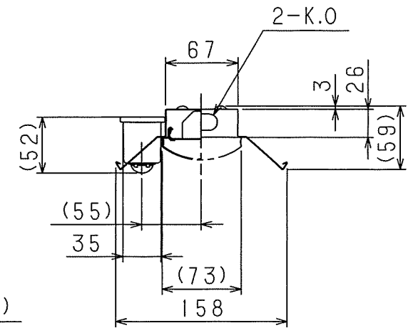
側面詳細図 (S=1:5)
