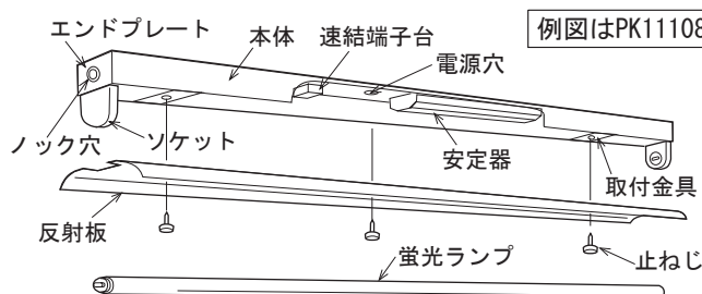
器具質量と背面取付穴（図1）
