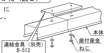
連結のしかた (図2)
