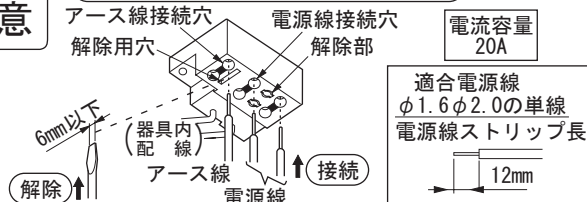
速結端子台の接続と解除 (図3)
