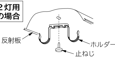
ランプの取り付けかた (図5)
