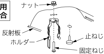
ホルダーの取り付けかた (図4)
