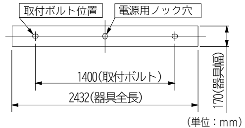
背面取付穴 (図1)
