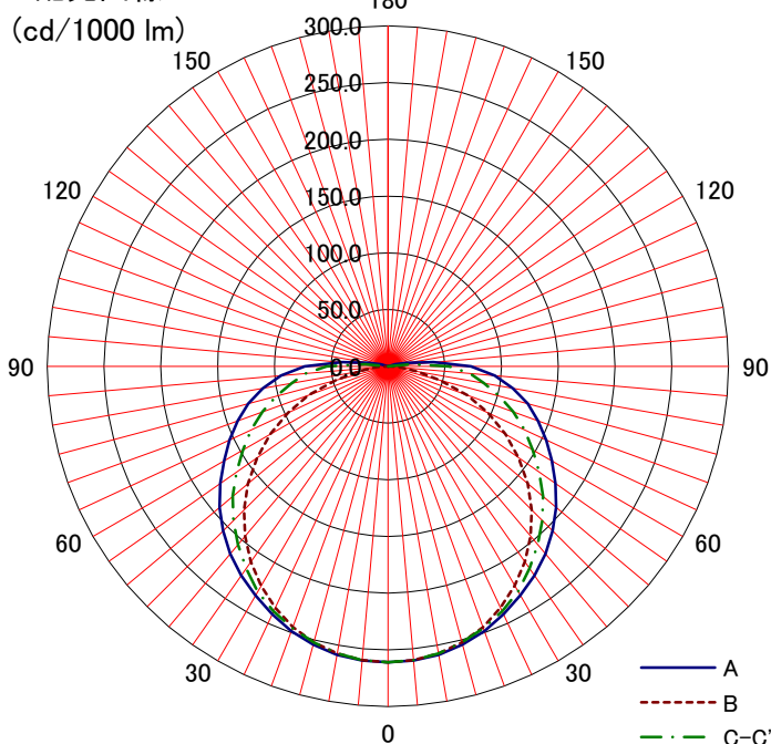
配光曲線
